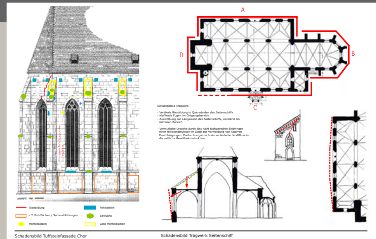
Ausschnitt Sanierungskonzept Stadtkirche Geislingen Steige
